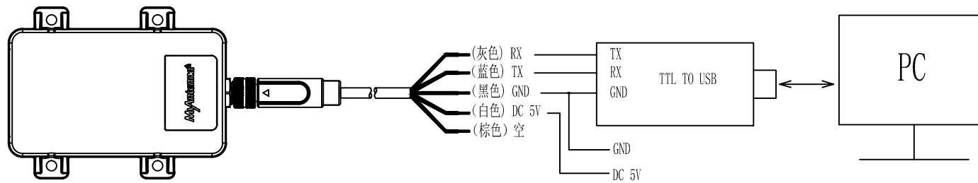
L1s传感器连接电脑图示
