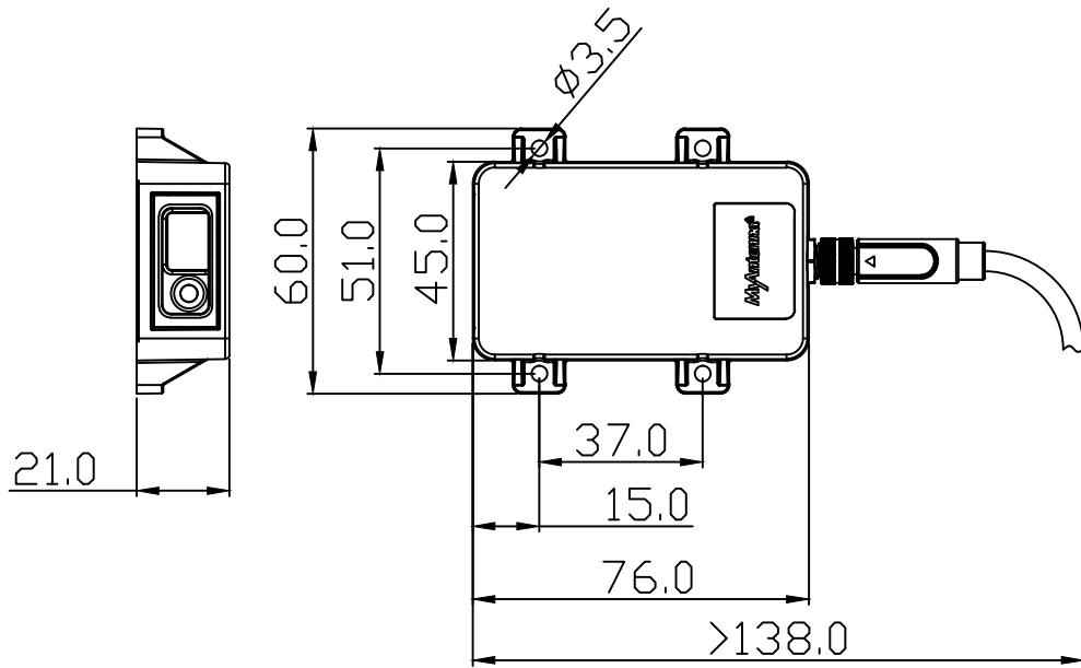
L1s传感器外形安装尺寸图
