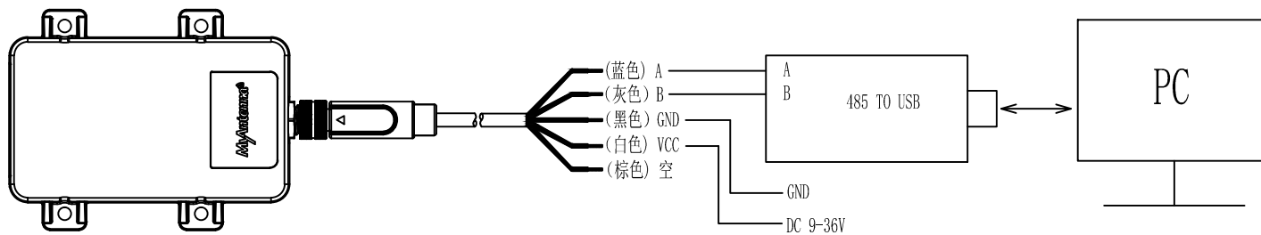
L2s传感器连接电脑图示
