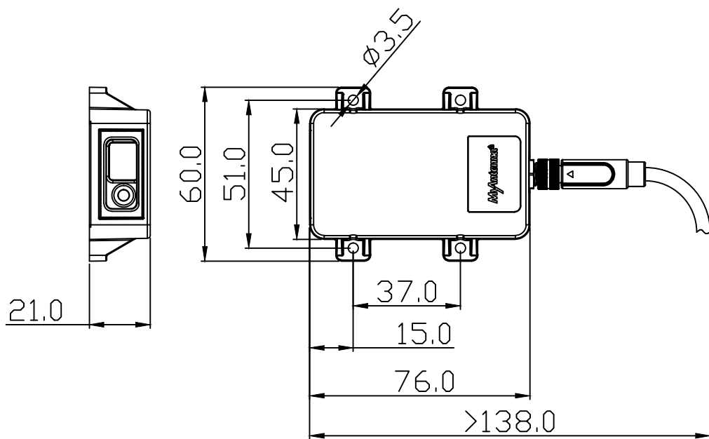
L2s传感器外形安装尺寸图
