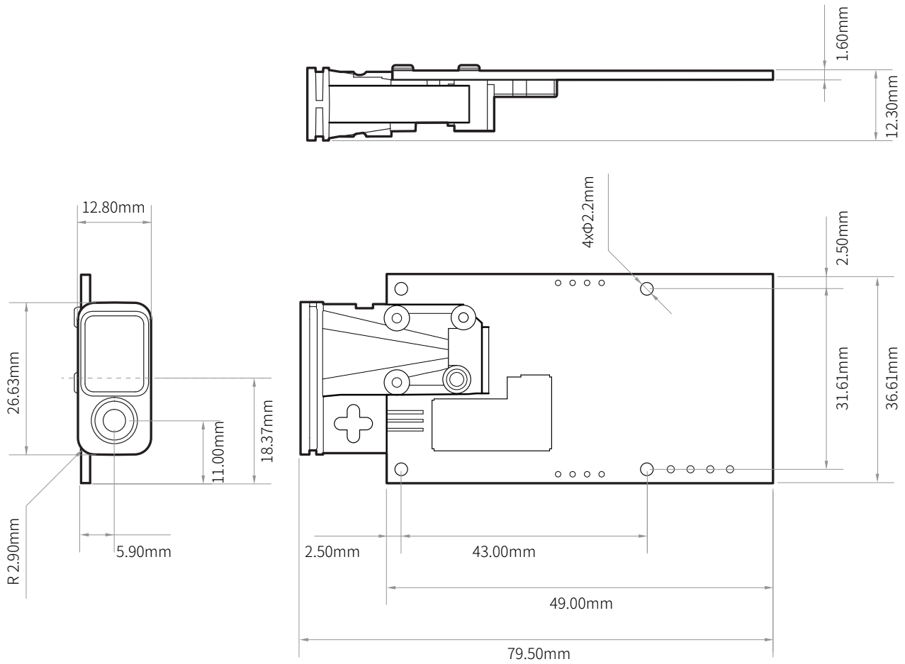
图 3. L3 尺寸图
