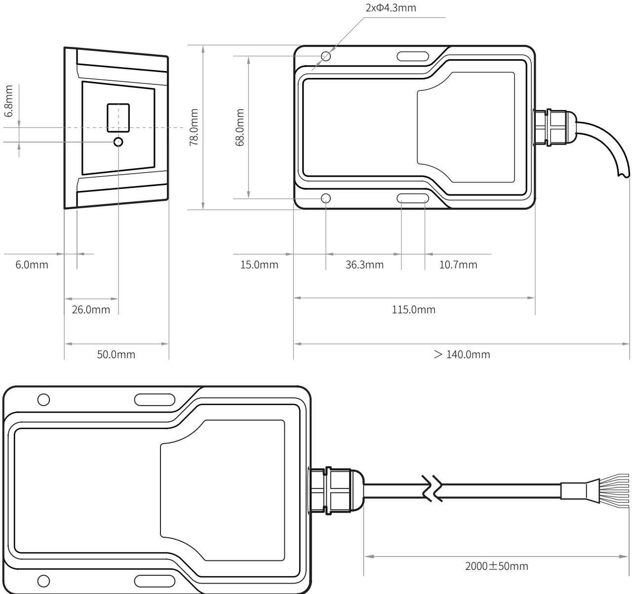
图 4. L3s/L3s-Filled 尺寸图
