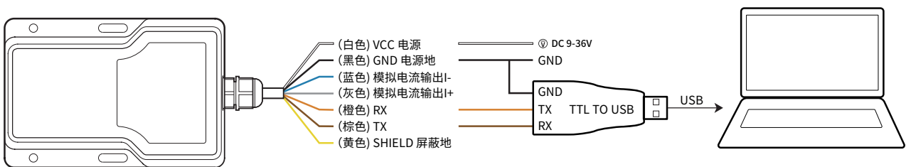
图 2. L3s/L3s-Filled 接线图
