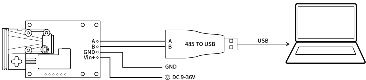
图 1. L2 接线图
