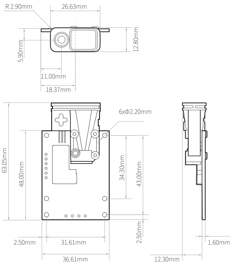
图 5. L2 尺寸图
