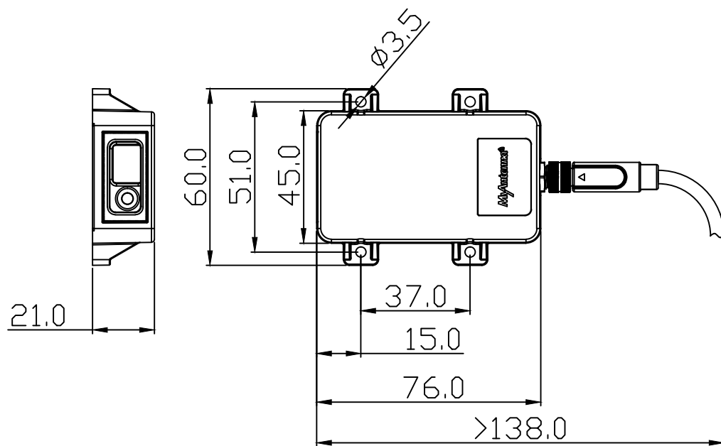
l4s传感器外形安装尺寸图
